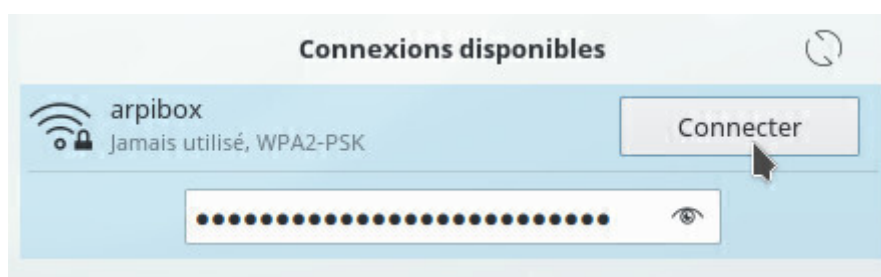
KDE : authentication
