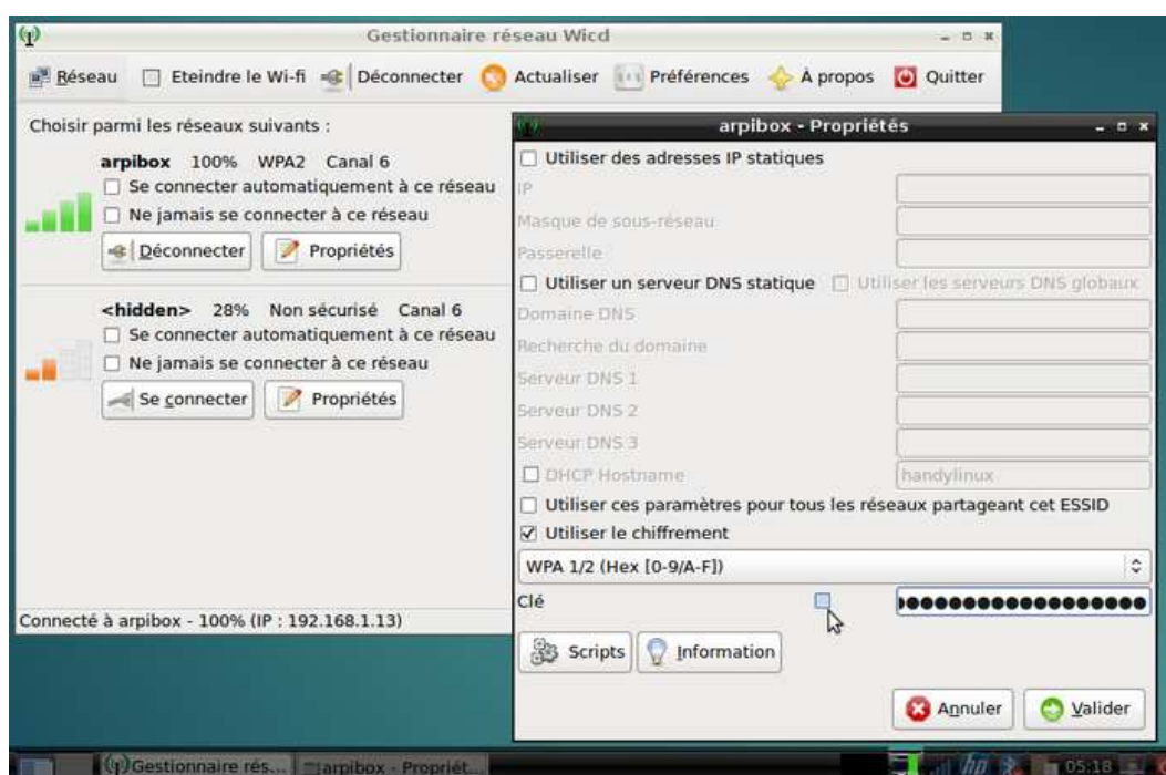
Wicd : propriétés de la connexion
