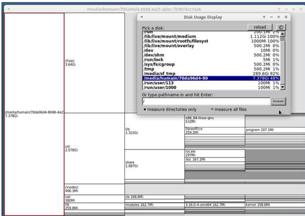
Xdiskusage en action
